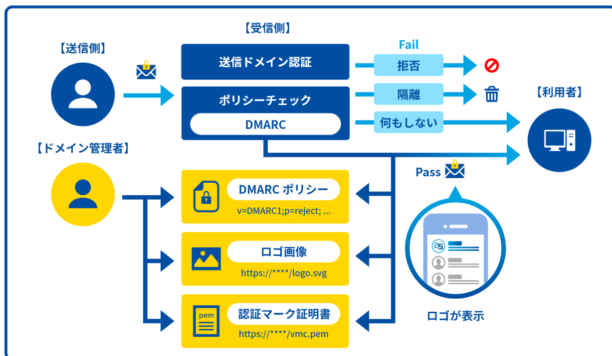
図. 送信側・受信側・利用者における BIMI の仕組み
